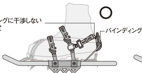
(図H) かかとにバイディングがあるアイゼンの固定方法
