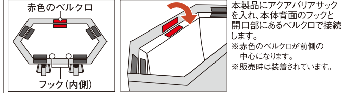
アクアバリアサックは高い防水性を誇りますが、水中などの水圧がかかる状況には適しません。荷物を満載した状態でアクアバリアサックを無理に抜かないでください。アクアバリアサックに負荷がかかり、破損する場合があります。
